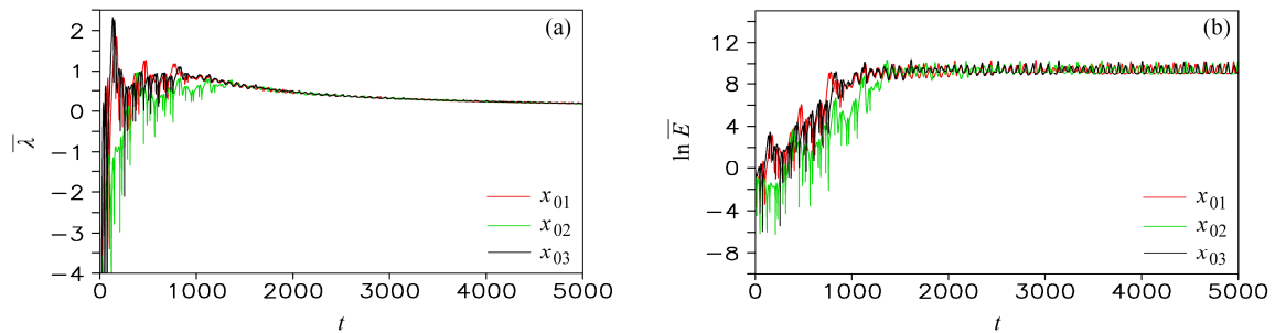
图 3 在 Lorenz63 系统里任选三个不同的初始状态 x_{01} 、 x_{02} 、 x_{03} ，在相同的初始误差域条件下，平均 NLLC ( \bar{\lambda}(x(t_0), \varepsilon) ) 以及局部平均误差相对增长 ( \bar{E}(x(t_0), \varepsilon) ) 的自然对数随时间 (无量纲) 的变化
