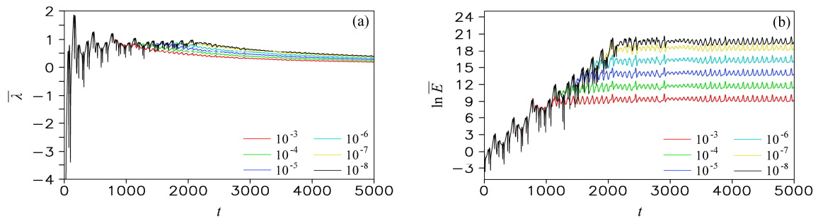
图 2 在 Lorenz63 系统里任选一个初始状态 x_{01} ，不同初始误差域条件下，平均 NLLC ( \bar{\lambda}(x(t_0), \varepsilon) ) 以及局部平均误差相对增长 ( \bar{E}(x(t_0), \varepsilon) ) 的自然对数随时间 (无量纲) 的变化。从上到下曲线对应的初始误差域分别为 10^{-8} 、 10^{-7} 、 10^{-6} 、 10^{-5} 、 10^{-4} 、 10^{-3}
