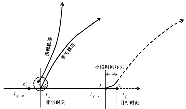
图 5 基于向前动力演化相似方法 (FLDA) 计算目标时刻 t_T 时的 LAGRE 方法示意图。此种情形下，目标状态 x_0 之后的时间序列未知， x_1 是 t_T 之前一小段时间 t_{T-si} 时刻的状态，通过局部动力演化相似方法确定 x_1 在历史资料里 t_{A-si} 时刻的相似状态 x'_1 ，进而确定 x_0 在相似时刻 t_A 时的相似状态 x'_0 ( t_T 和 t_{T-si} 间隔很小)，计算 t_A 时刻的 LAGRE 代替 t_T 时刻的 LAGRE
