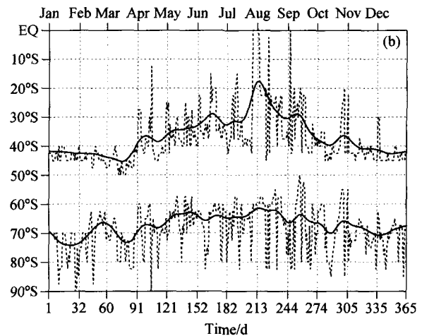
图 1 1948~2005 年北半球 (a) 和南半球 (b) 逐日纬向平均 SLP 各纬度之间交叉相关中最大负相关系数相对的两个纬度的年变化。粗实线: 31 天 Gauss 平滑序列
