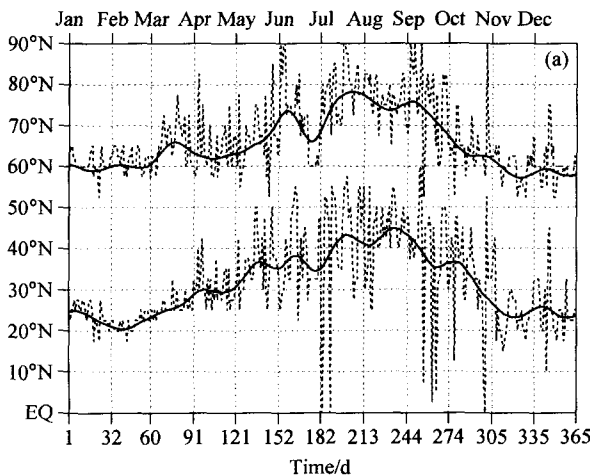
图 1 1948~2005 年北半球 (a) 和南半球 (b) 逐日纬向平均 SLP 各纬度之间交叉相关中最大负相关系数相对的两个纬度的年变化。粗实线: 31 天 Gauss 平滑序列
