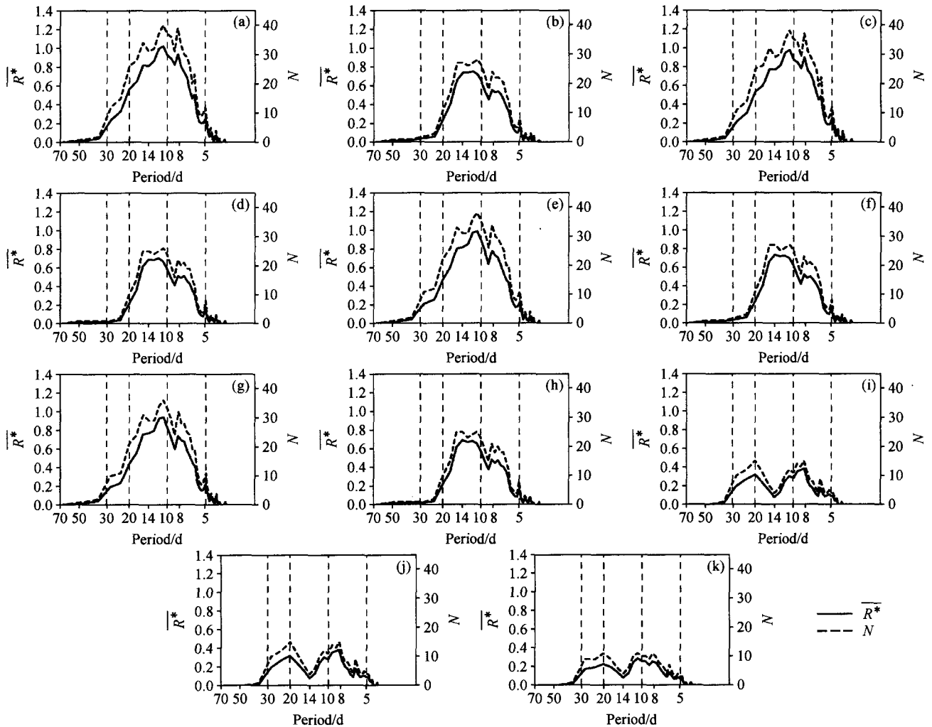
图5 1948~2005年NAMI全年(365天)标准化功率谱 \overline{R^*} 合成及对应周期上功率谱通过显著性检验的年份总数统计 N : (a) 所有年份; (b) 所有不含准3W的年份; (c) 所有含准1W的年份; (d) 含准1W、无准3W的年份; (e) 所有含准2W的年份; (f) 含准2W、无准3W的年份; (g) 既有准1W又有准2W的所有年份; (h) 既有准1W又有准2W年份, 但无准3W的年份; (i) 含有准3W的所有年份; (j) 既有准1W又有准3W的所有年份; (k) 既有准2W又有准3W的所有年份
