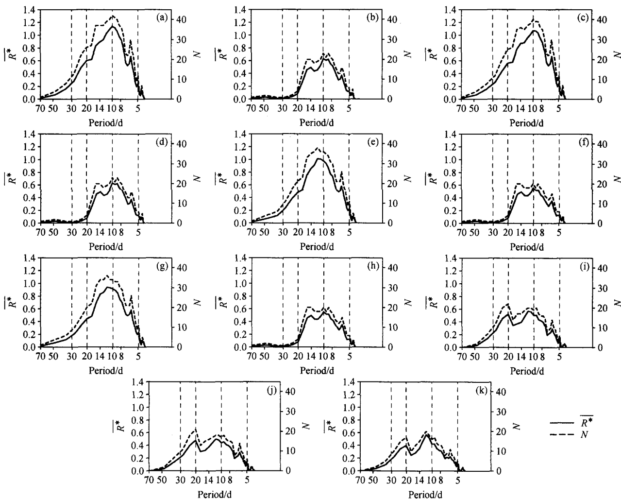
图8 同图5, 但为 SAMI 全年 (365 天)
