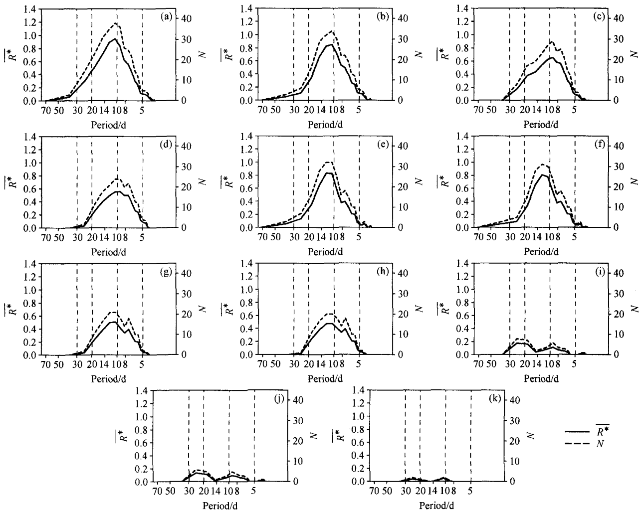
图6 同图5, 但为MAMI活跃期(11~3月)
