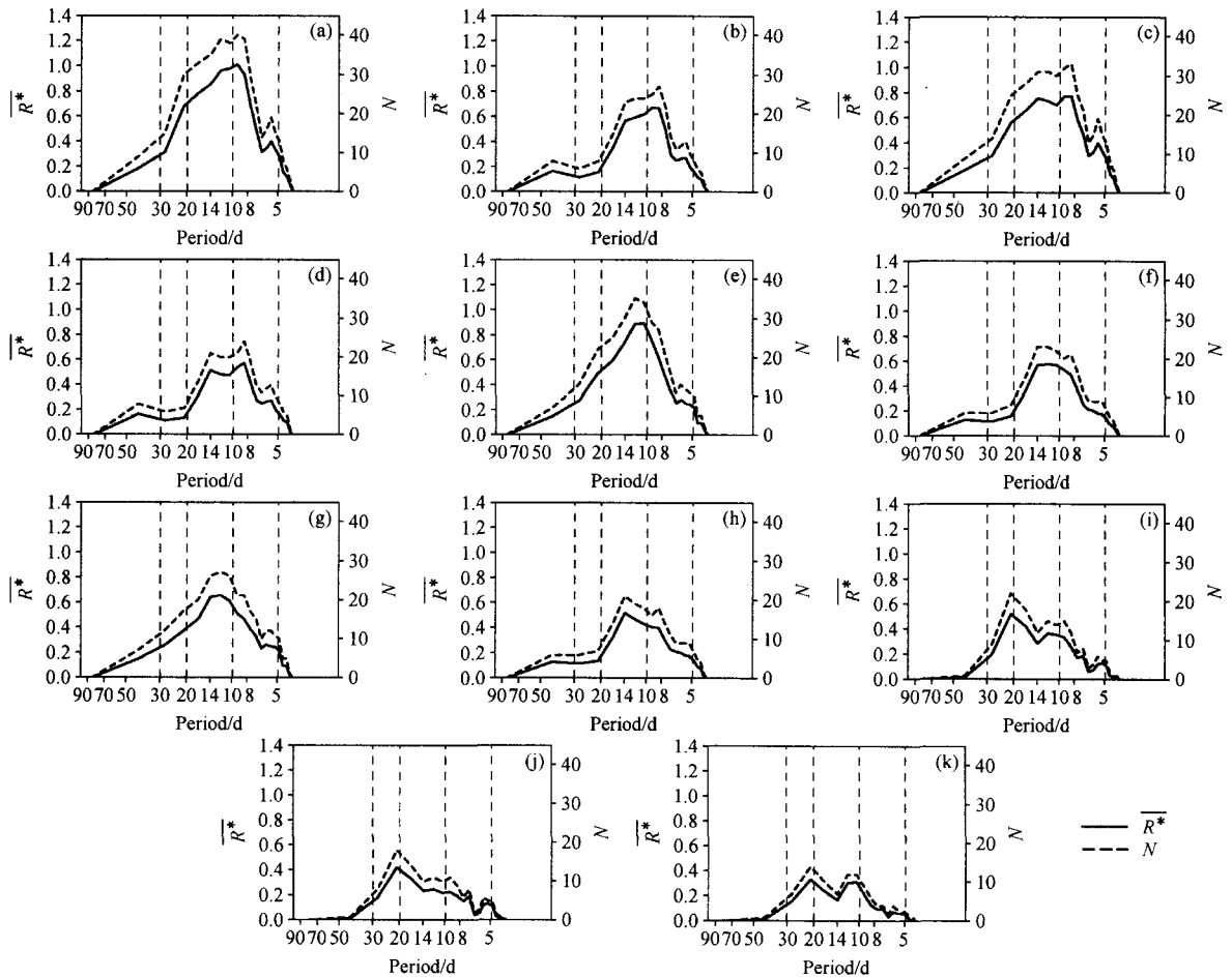
图 10 同图 5, 但为 SAMI 后半年 (7~12 月)
