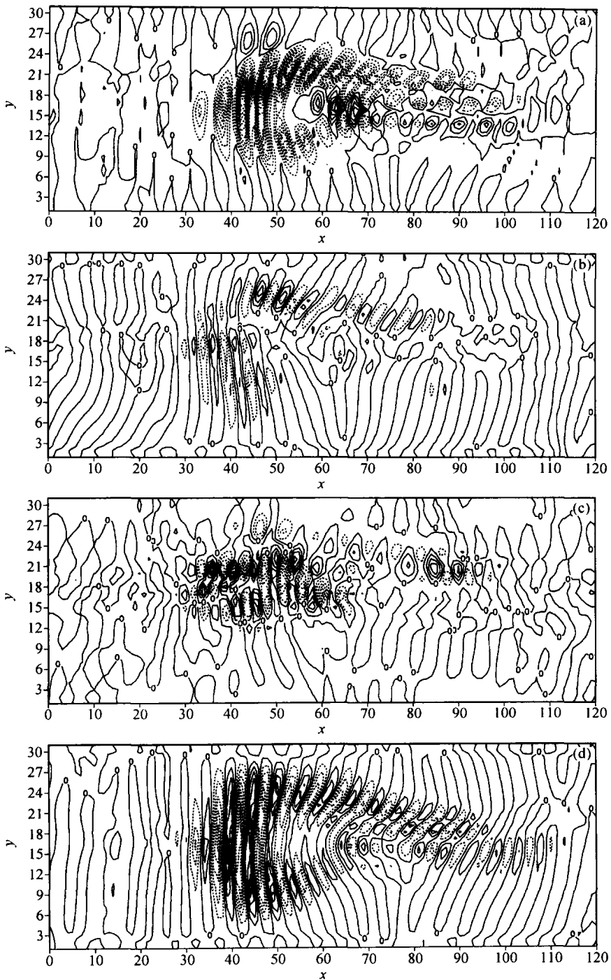
图 10 地形强迫下“ ”型阻塞积分第 44 天瞬变扰动能量变化分布，实线为正值，虚线为负值 (a) 背景流能量向扰动流场转换（等值线间距为 0.02）；(b) 背景流场平流作用对局地扰动场的贡献（等值线间距为 0.1）；(c) 非地转气压扰动通量在局地的辐散辐合（等值线间距为 0.05）； (d) 总扰动能量变化趋势（等值线间距为 0.1）
