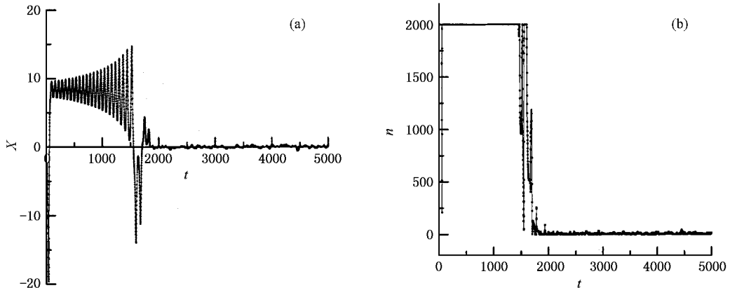
图 1 初值集合处在 (-0.5, -0.5, 0.5) 附近, Lorenz 系统的平均预报 X 分量和落入动态窗口中的粒子数 n 随积分时间 t (即迭代步数,下同)的演化图 (a)平均预报 X 分量 (b)落入动态窗口中的粒子数 n
